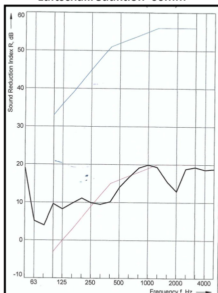
Luftschallreduktion 60mm
